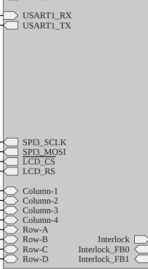
U_Microcontroller Microcontroller.SchDoc
